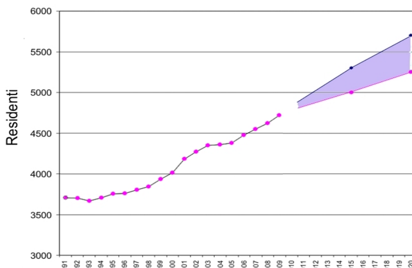
Villa d'Adda - Andamento della popolazione residente dal 1991 e previsioni al 2015 e 2020
